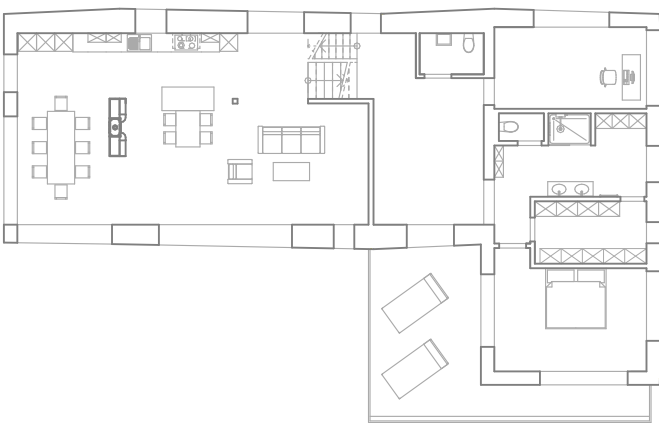
REZ-DE-CHAUSSEE
